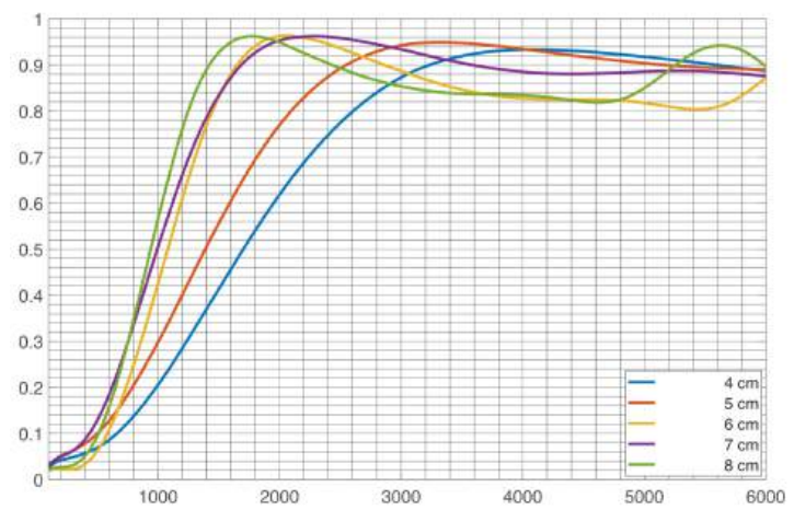
Simulace koeficientu absorpce zvuku s Thomassonovou korekcí
